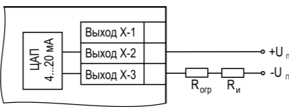
Рисунок 20 – Схема подключения нагрузки к ВУ типа И
