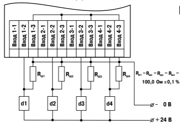
Рисунок 8 – Пример схемы подключения активных датчиков d1-d4 с выходным сигналом тока от 4 до 20 mA
