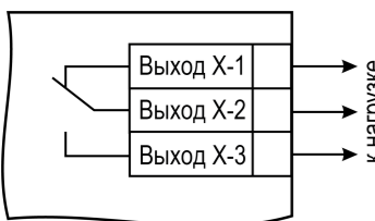
Рисунок 11 – Схема подключения нагрузки к ВУ типа Р
