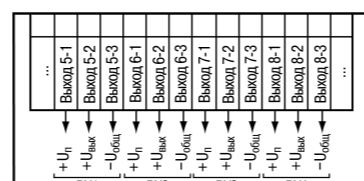
Рисунок 22 – Схема подключения выходных устройств прибора TRM 13x-U
