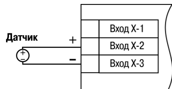
Рисунок 9 – Схема подключения активного датчика с выходом в виде напряжения 0...+50 мВ или 0...1 В
