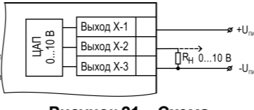
Рисунок 21 – Схема подключения нагрузки к ВУ типа У
