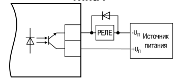
Рисунок 13 – Схема подключения нагрузки к ВУ типа К
