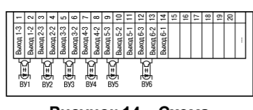
Рисунок 14 – Схема подключения транзисторных оптопар прибора TRM136-К
