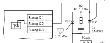
Рисунок 16 – Схема встречно-параллельного подключения двух тиристоров к ВУ типа С
