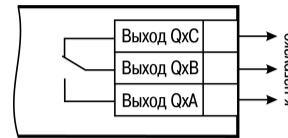
Рисунок 9 – Схема подключения нагрузки к ВЭ типа «Р»
