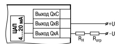
Рисунок 15 – Схема подключения нагрузки к ВЭ типа «И»
