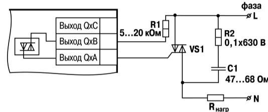
Рисунок 11 – Схема подключения силового симистора к ВЭ типа «С»
