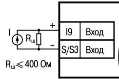
Рисунок 7 – Схема подключения активного датчика с выходом типа «Ток 4...20 мА» (к входам I10–I12 аналогично)
