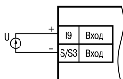
Рисунок 6 – Схема подключения активных датчиков с выходом типа «Напряжение 0...10 В» (к входам I10–I12 аналогично)
