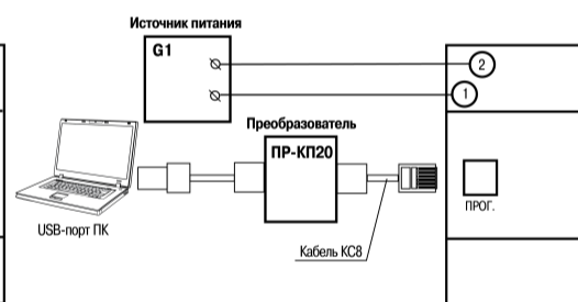
Рисунок 17 – Схема подключения к ПК (через преобразователь ПР-КП20)
