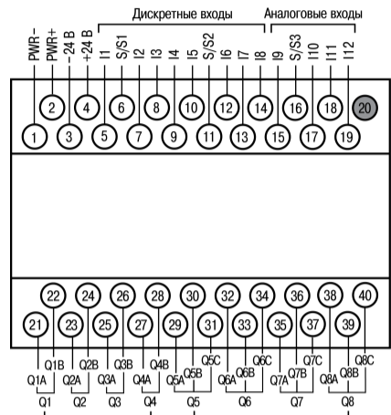
Рисунок 3 – Расположение контактов
