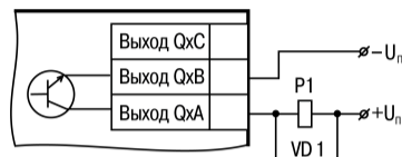
Рисунок 10 – Схема подключения нагрузки к ВЭ типа «К»
