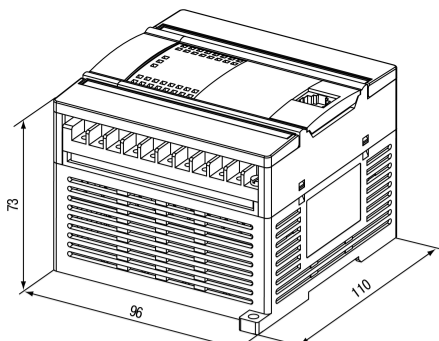
Рисунок 1 – Габаритный чертёж
