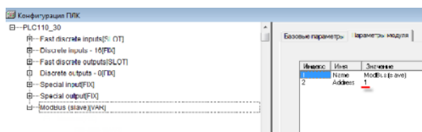
Рисунок 13.4 – Добавление и настройка элемента Modbus (Slave)
