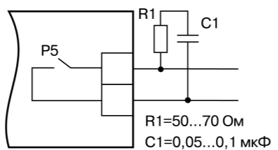
Рисунок 11 – Схема подключения нагрузки к ВУ типа P
