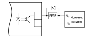
Рисунок 13 – Схема подключения нагрузки к ВУ типа K
