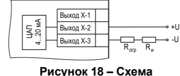
Рисунок 18 – Схема подключения нагрузки к ВУ типа И
