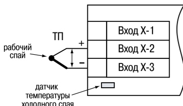
Рисунок 7 – Схема подключения терморпары
