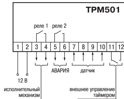
Рисунок 5.1 – Контакты клеммника
