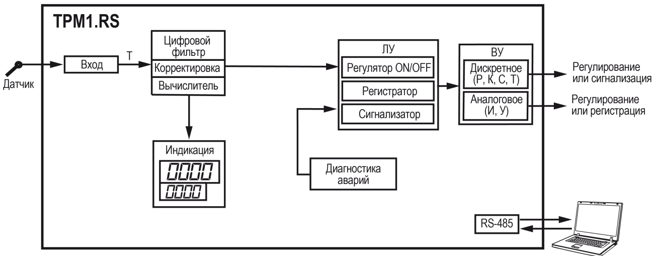
Рисунок 6.1 – Функциональная схема
