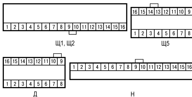
Рисунок 7.7 – Установка переключки
