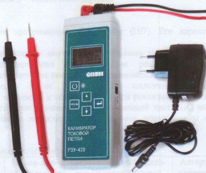
Рисунок 2 - Общий вид прибора с адаптером питания и подключенными измерительными выводами (щупами)
