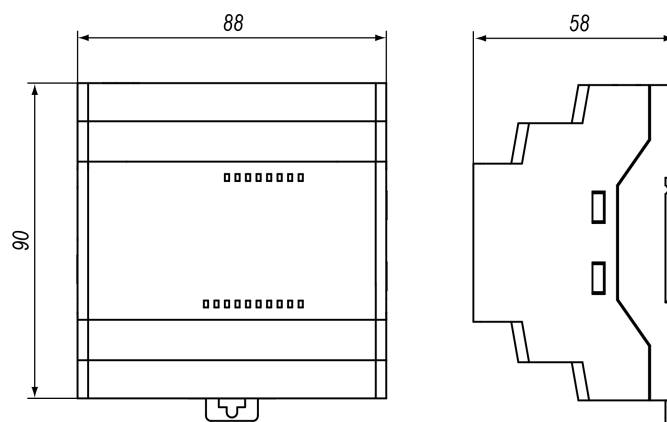
Рисунок 5.1 – Габаритные размеры
