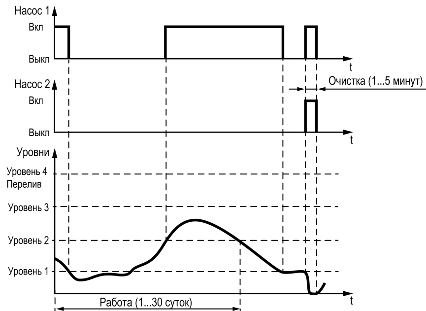
Рисунок 9.3 – Очистка от стоков
