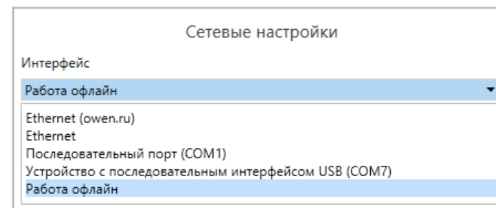
Рисунок 4.3 – Добавление устройства
