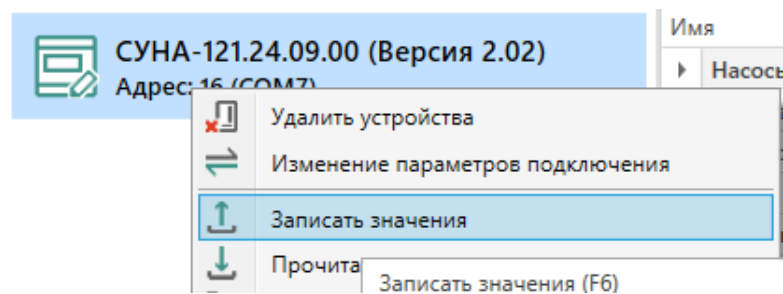
Рисунок 4.16 – Контекстное меню
