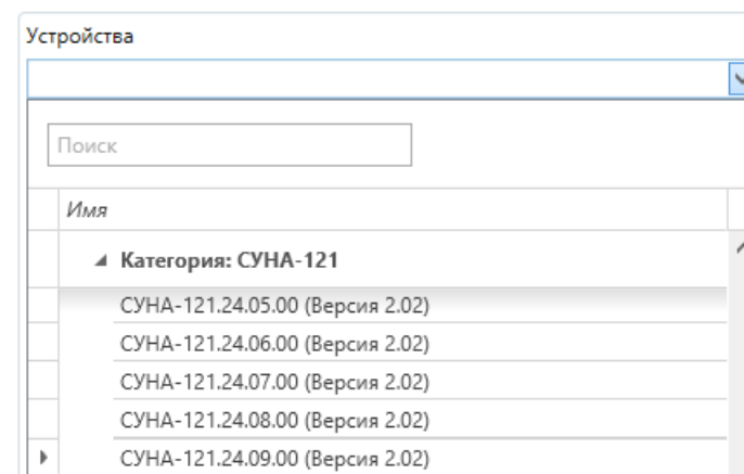
Рисунок 4.4 – Выбор модификации
