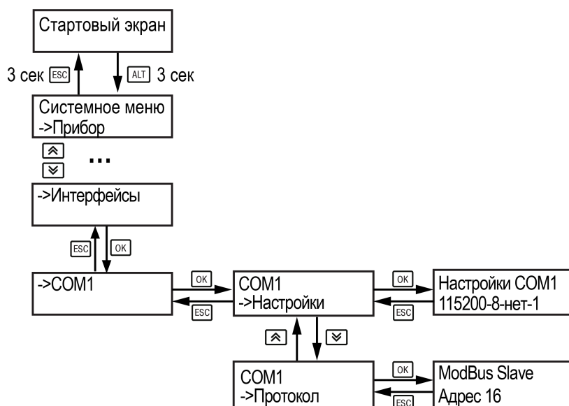
Рисунок 11.1 – Настройка параметров сетевого интерфейса
