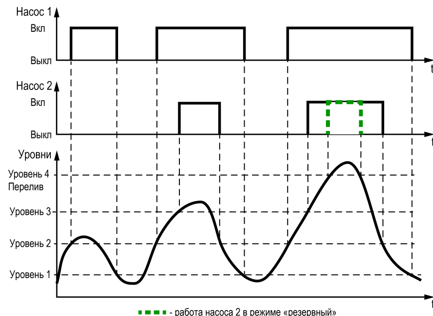
Рисунок 9.1 – Регулирование уровня
