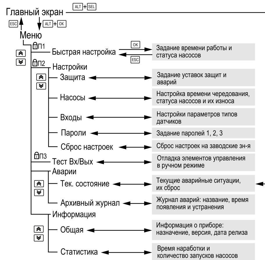
Рисунок 7.2 – Схема переходов по меню
