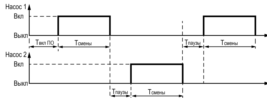
Рисунок 9.2 – Чередование насосов
