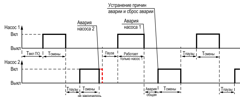
Рисунок 9.6 – Авария насосов
