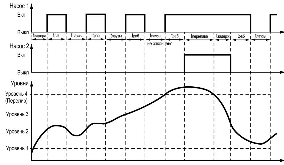
Рисунок 9.5 – Авария аналогового датчика уровня
