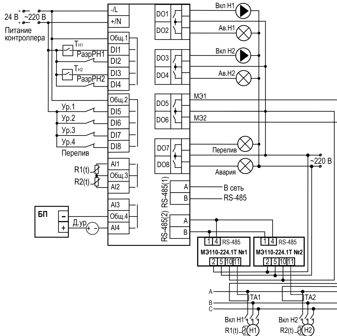
Рисунок 5.4 – Схема подключения СУНА-121.X.09.00
